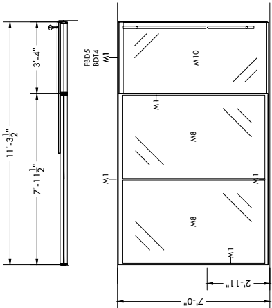
1 ELEVATION A SCALE: 1/4" = 1'-0"
