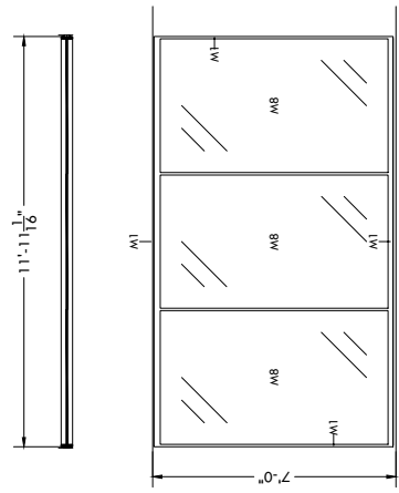
3 ELEVATION C SCALE: 1/4" = 1'-0"
